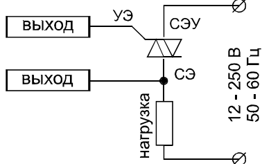
Рис.2. Схема подключения симисторов ТС122-25, ТС142-80.
